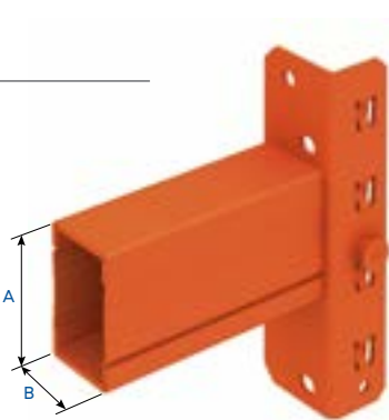
Larguero 2C-S (1115) Formado por dos perfiles en forma de C encajados uno dentro del otro y soldados a una grapa.
