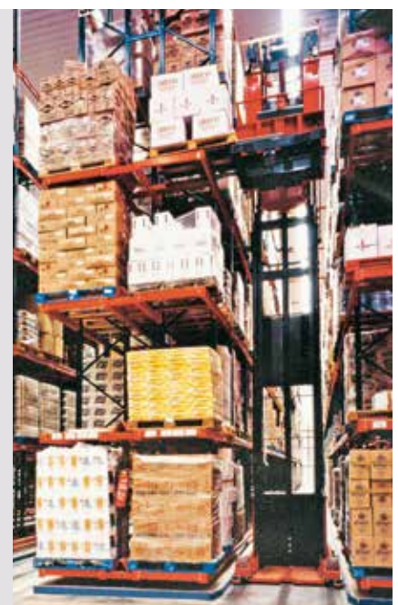
Horquilla bilateral
