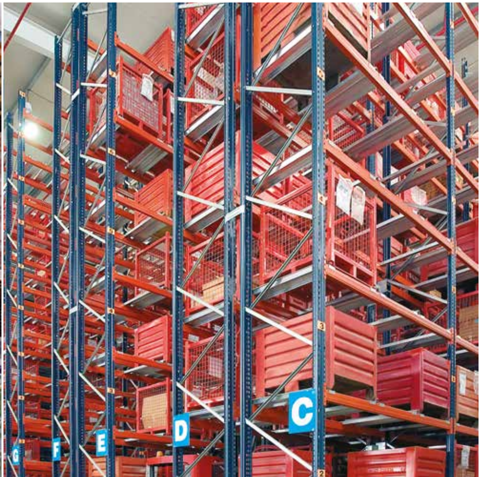
Almacén de paletización convencional con contenedores metálicos
