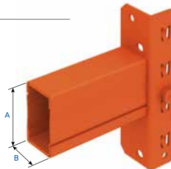
Larguero 2C-S (1115) Formado por dos perfiles en forma de C encajados uno dentro del otro y soldados a una grapa.
