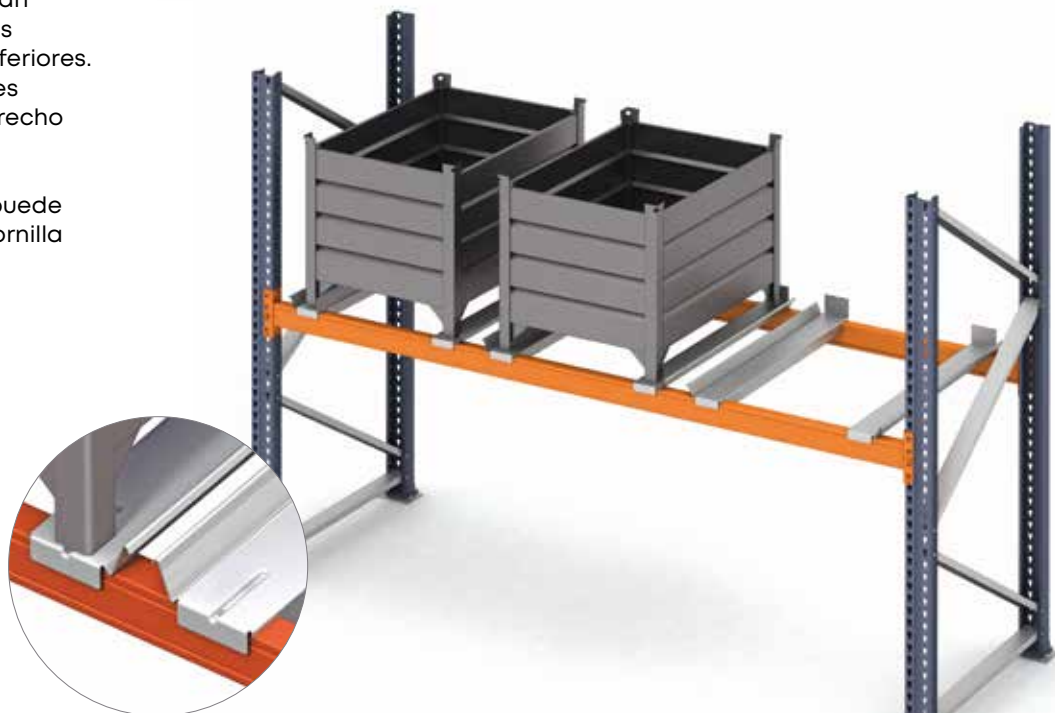
Tope para el soporte contenedor
