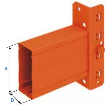
Larguero TB (100, 120, 130)
