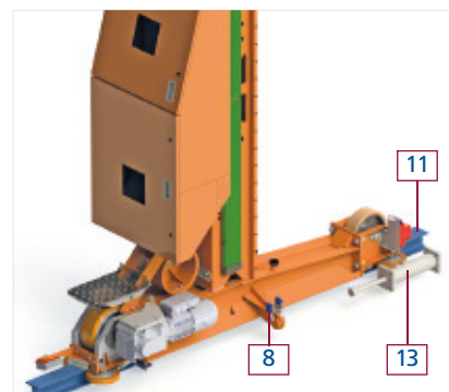
Carril inferior (11), tope hidráulico de final de recorrido (13) y telémetro (8).
