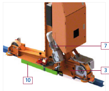
Testero inferior (3), toma de corriente (10) y equipo de elevación (7)
