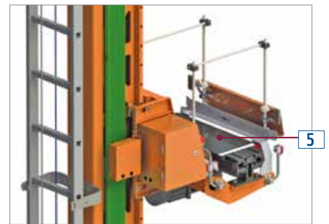
Cuna o bastidor móvil de elevación (5).
