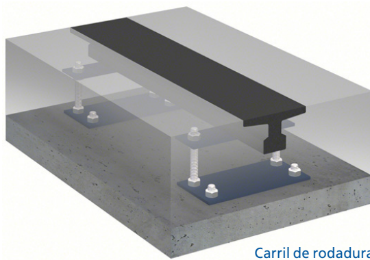
Carril guía
